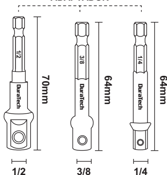
ADAPTADOR
