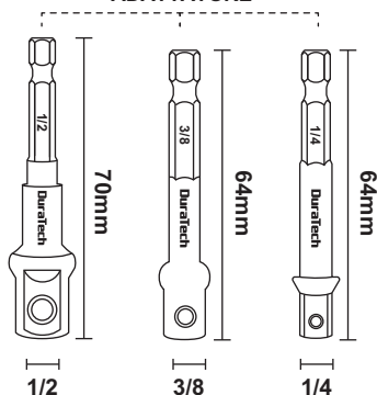
ADATTATORE
